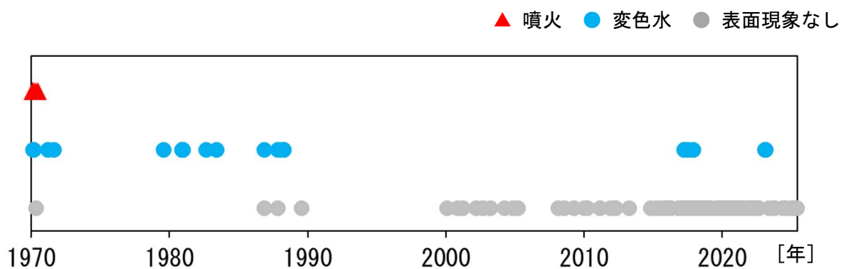
図4 ベヨネース列岩 1970年以降の活動状況
