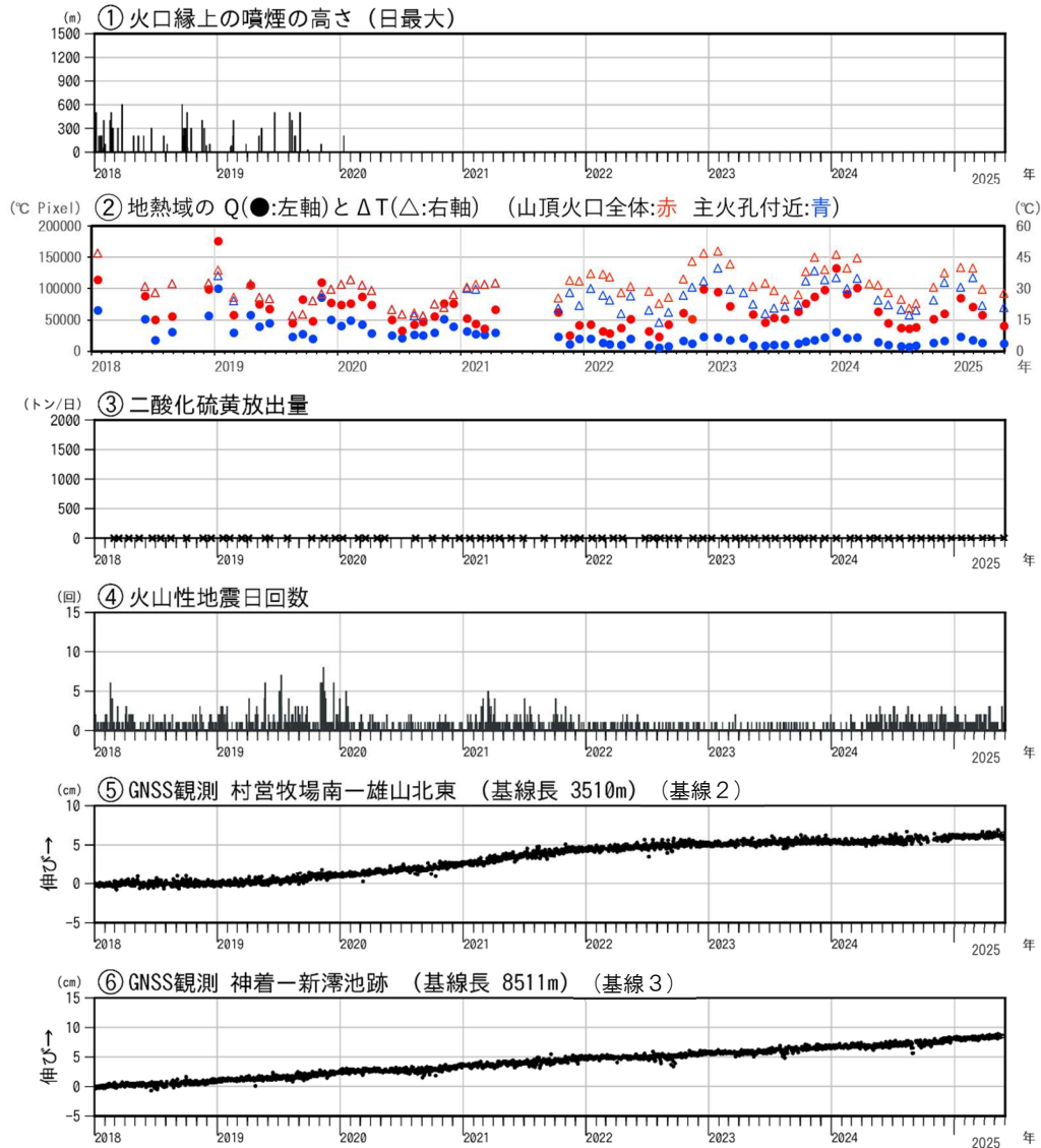
図6 三宅島 火山活動経過図（2018年1月1日～2025年5月31日）
