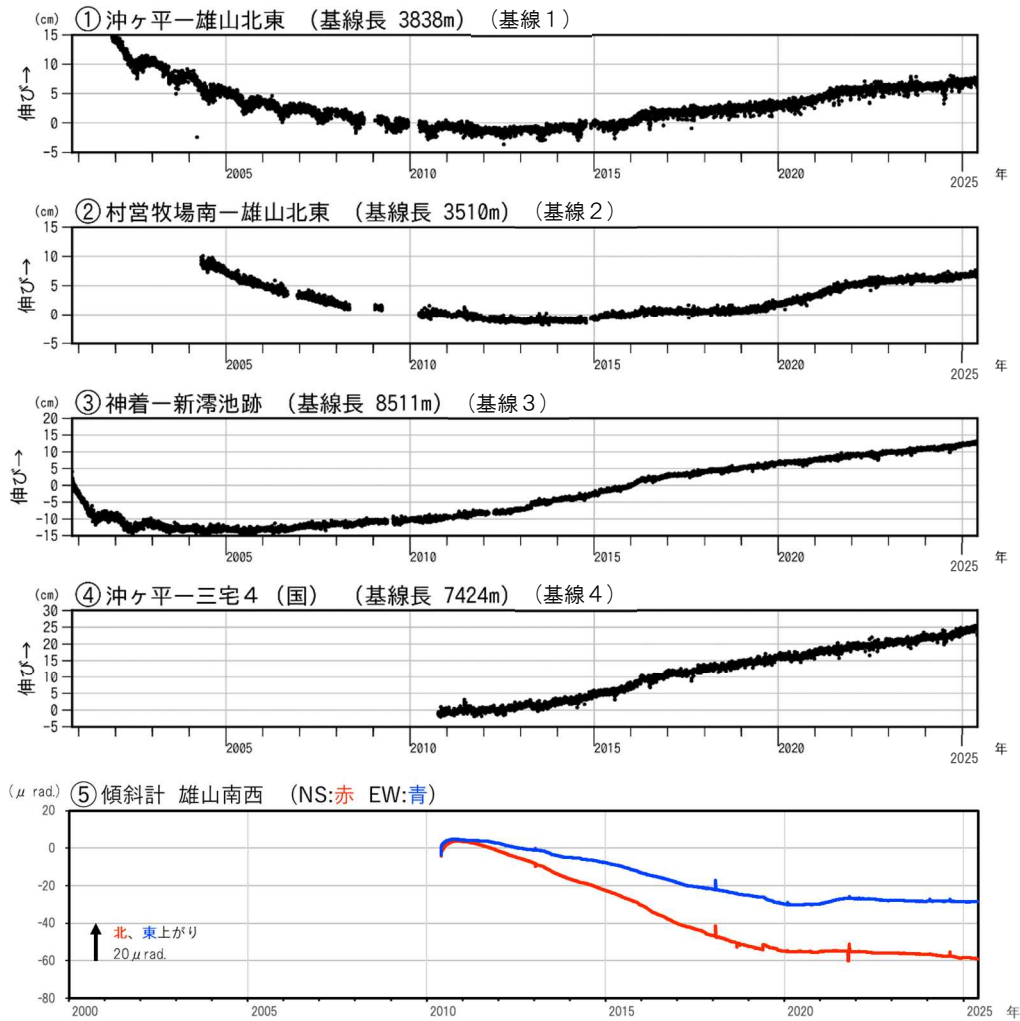
図8 三宅島 GNSS 連続観測及び傾斜計観測結果（2000 年 10 月 26 日～2025 年 5 月 31 日）
