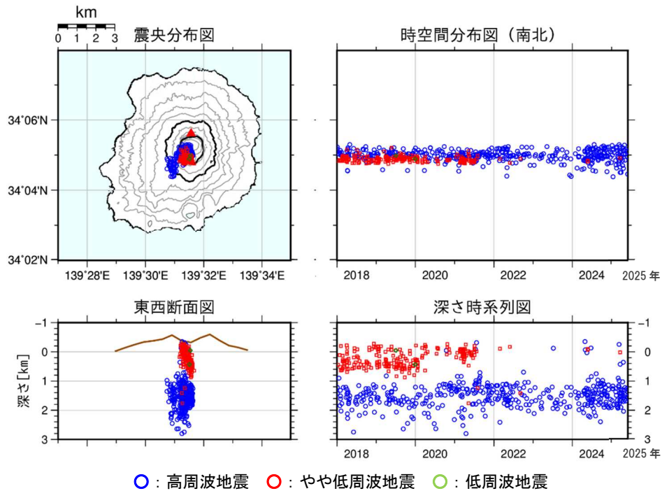
図 9 三宅島 震源分布図
