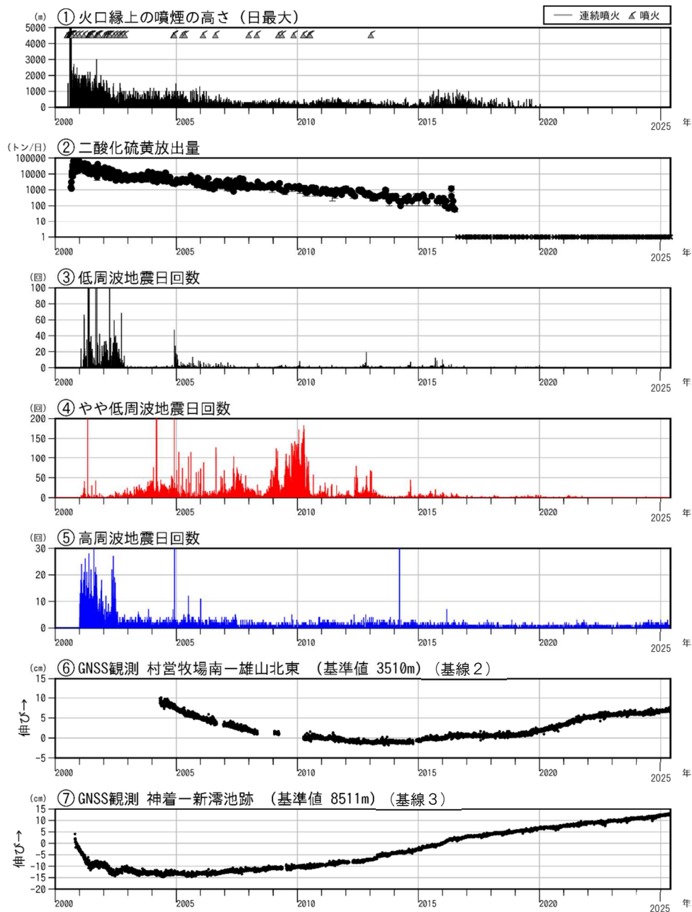
図7 三宅島 長期の火山活動経過図（2000年1月1日～2025年5月31日）
