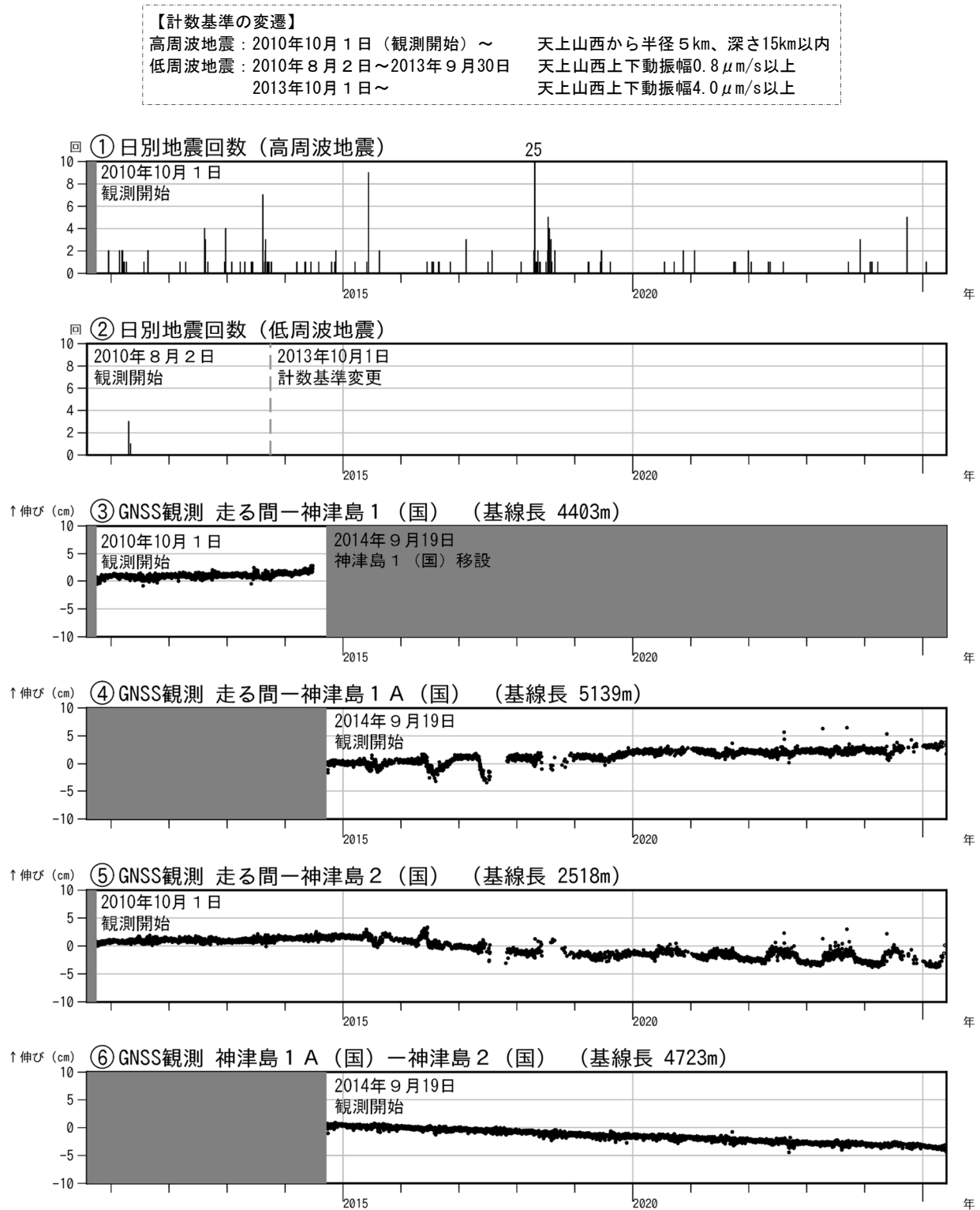
図2 神津島 火山活動経過図(2010年8月2日～2025年5月31日)
