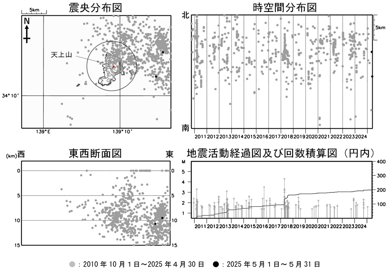
図3 神津島 広域地震観測網による山体・周辺の地震活動（2010年10月1日～2025年5月31日） 広域地震観測網により震源決定したもので、深さは全て海面以下として決定しています。なお、2020年9月以降については、地震観測点の標高を考慮する等、震源決定の手法を変更しています。 M（マグニチュード）は地震の規模を表し、M1.4以上の地震を示しています。 図中の震源要素は一部暫定値が含まれており、後日変更することがあります。 計数対象（天上山西から半径約5km、深さ約15km以内）以外の地震が含まれるため、図2-①の日別地震回数（高周波地震）とは異なります。 震央分布図中の円は火山性地震の回数の計数対象（天上山西から半径5km、深さ15km以内）の範囲を示しています。 ・地震活動は低調に経過しました。
