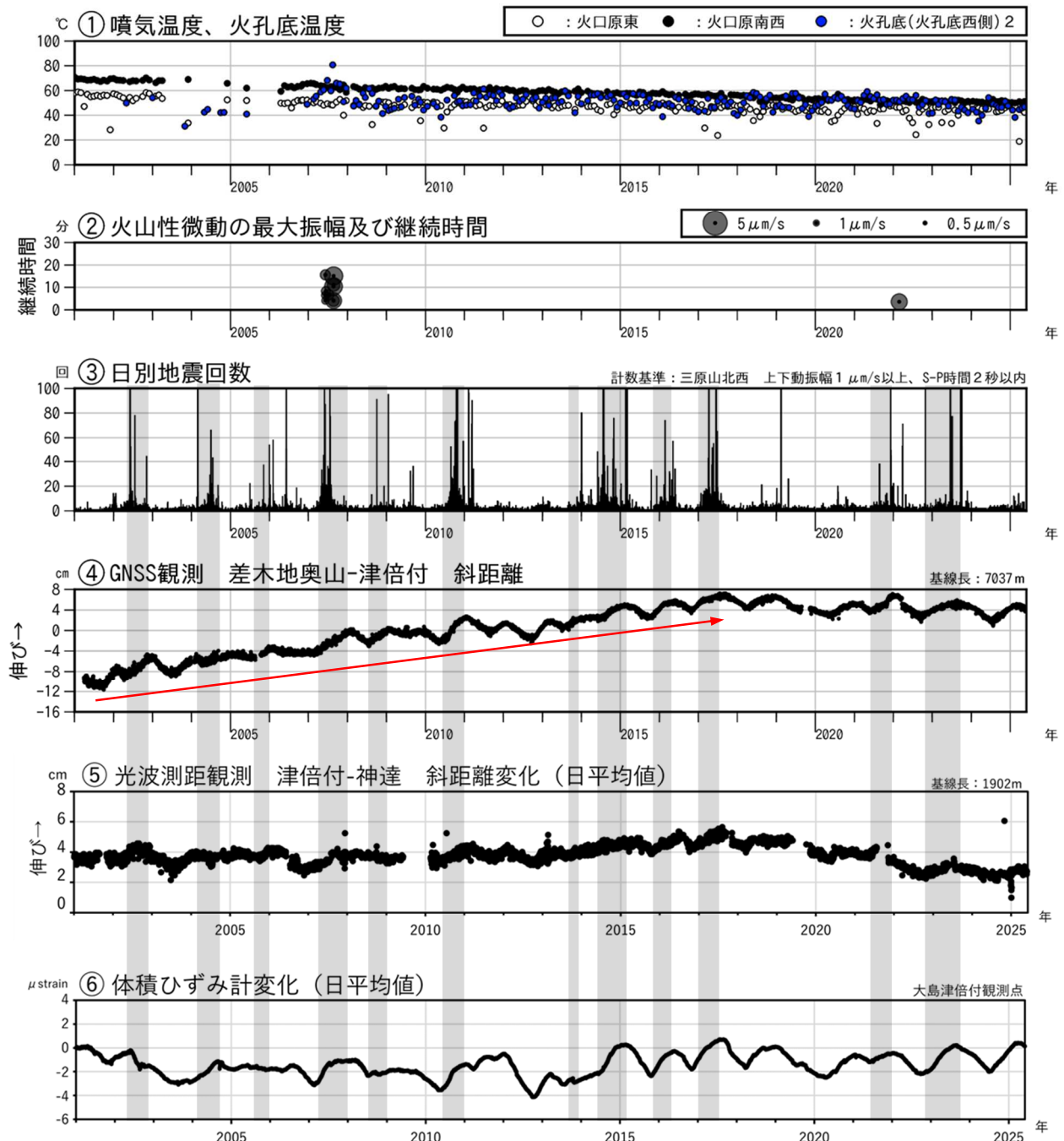
図2 伊豆大島 最近の火山活動経過図（2001年1月～2025年5月31日）
