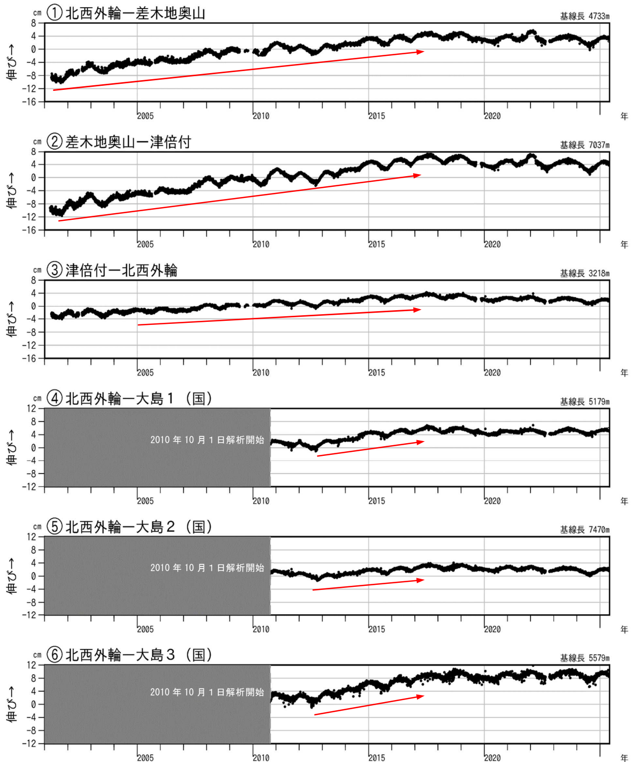
図 3-1 伊豆大島 GNSS 連続観測による基線長変化(2001 年 1 月～2025 年 5 月 31 日)
