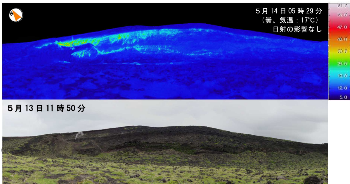
図7-2 伊豆大島 剣ガ峰の状況（撮影方向は図8参照）
