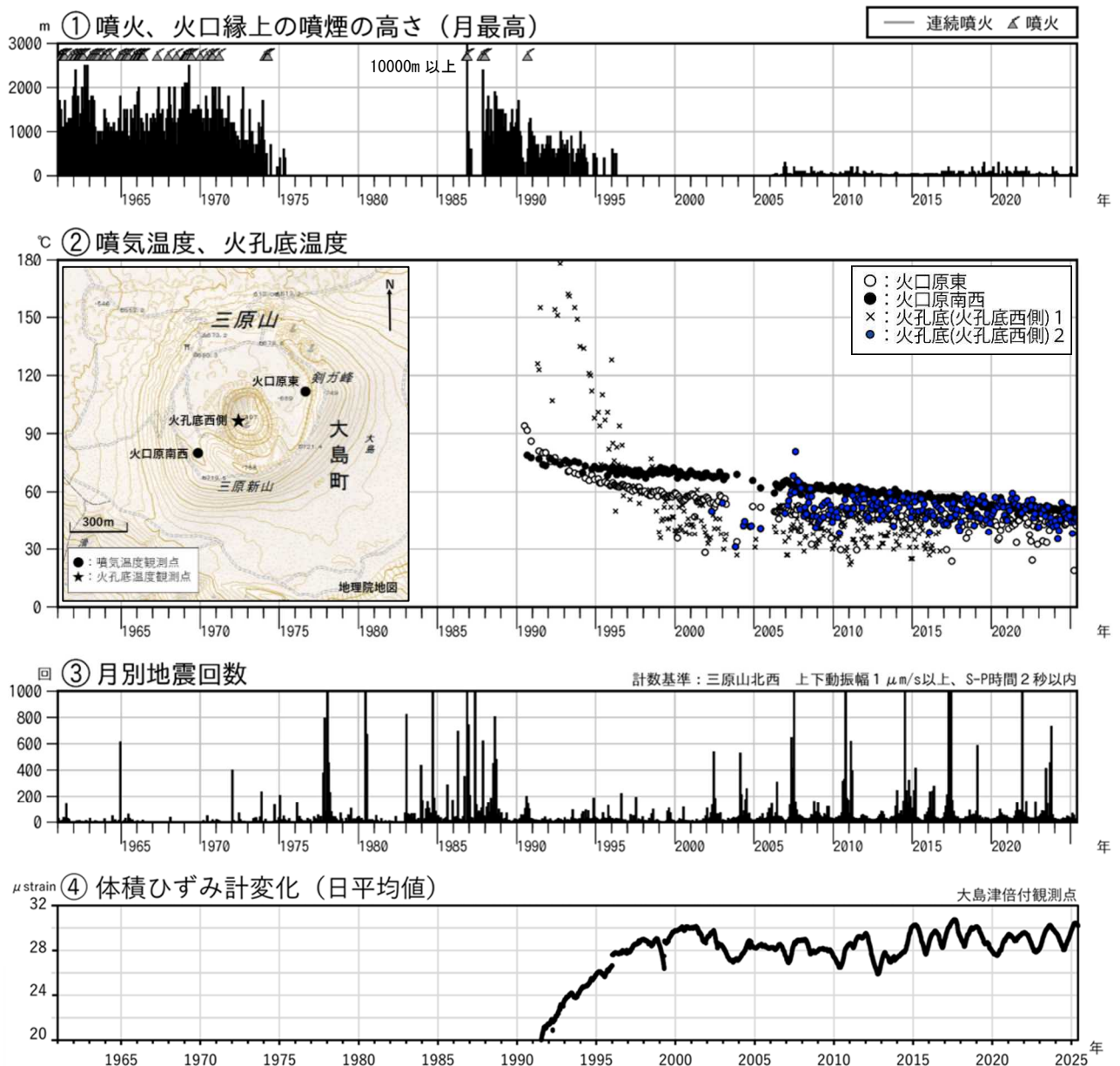
図1 伊豆大島 長期間の火山活動経過図（1961年1月～2025年5月31日）
