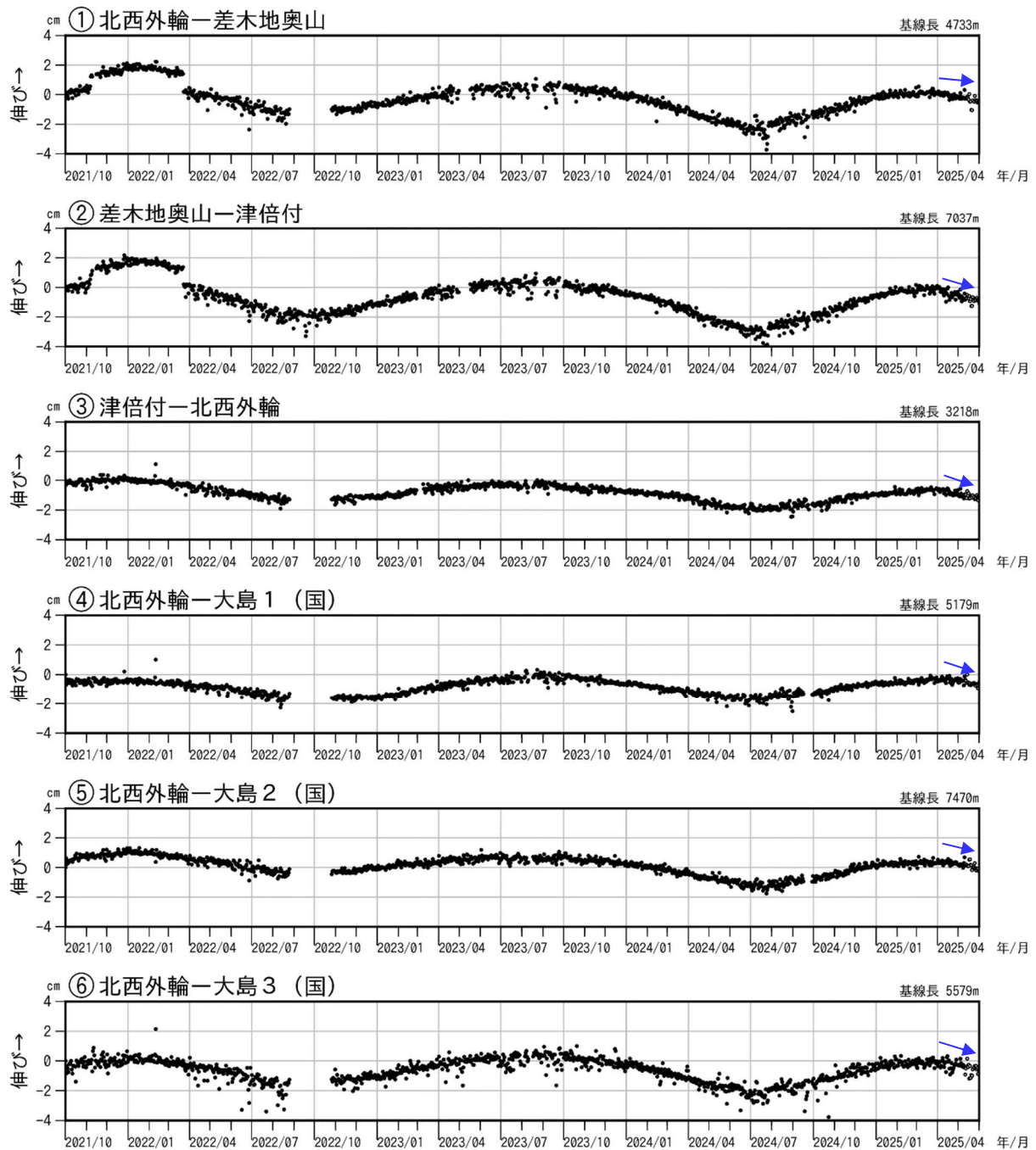
図 3-2 伊豆大島 GNSS 連続観測による基線長変化 (2021 年 10 月～2025 年 5 月 31 日)
