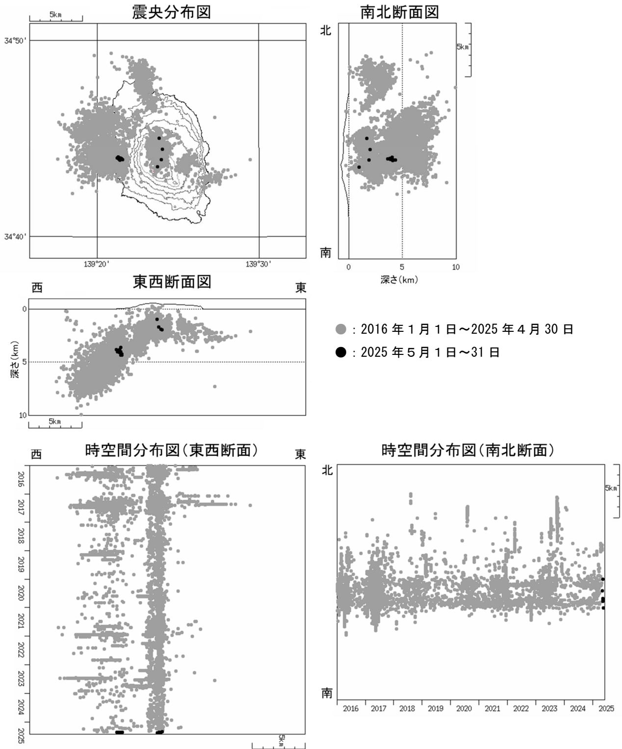
図4 伊豆大島 震源分布図（2016 年 1 月 1 日～2025 年 5 月 31 日）
