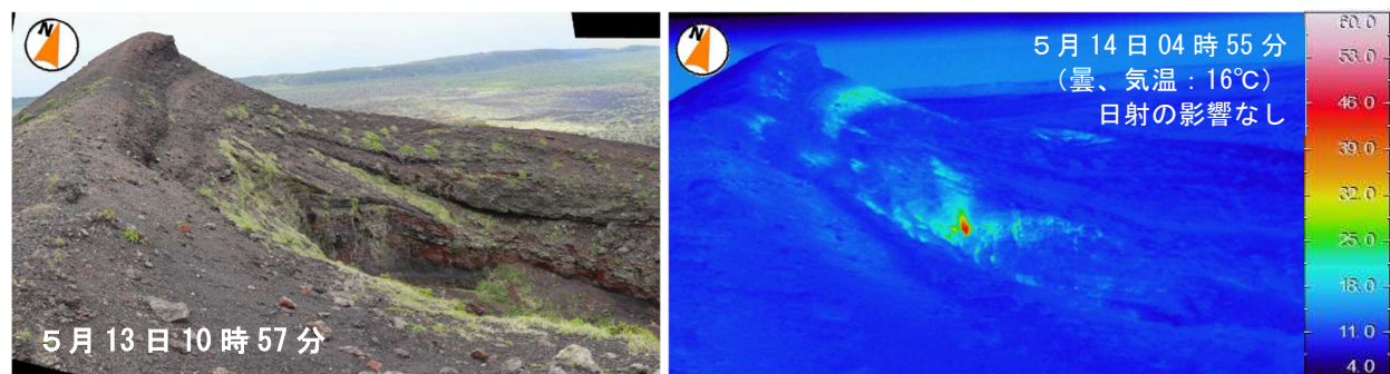
図7-1 伊豆大島 B2 火孔周辺の状況（撮影方向は図8参照）
