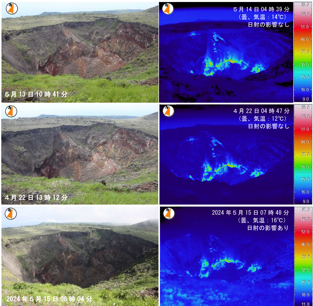
図6 伊豆大島 中央火孔内の状況（撮影方向は図8参照）
