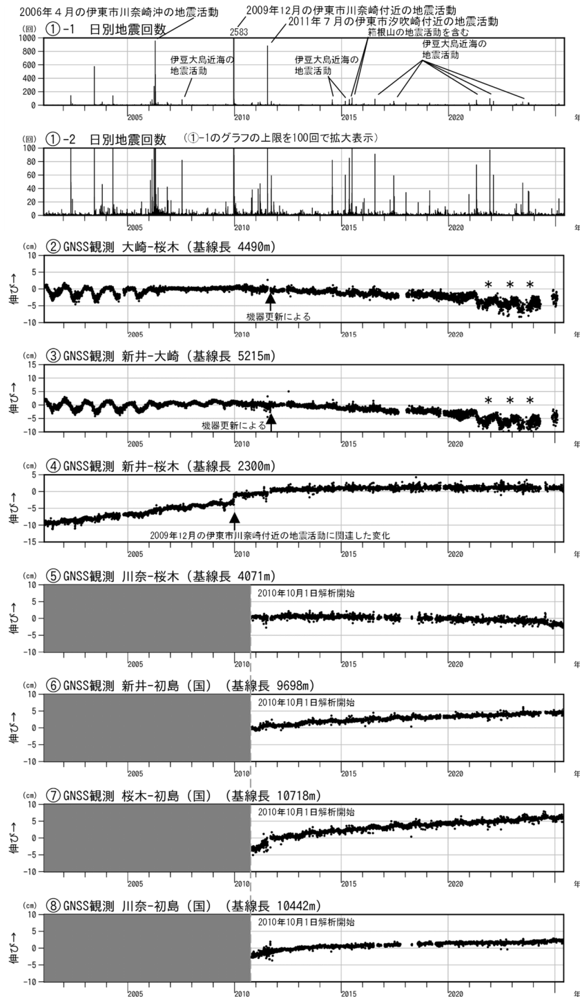
図3 伊豆東部火山群 火山活動経過図（2001年2月1日～2025年5月31日）
