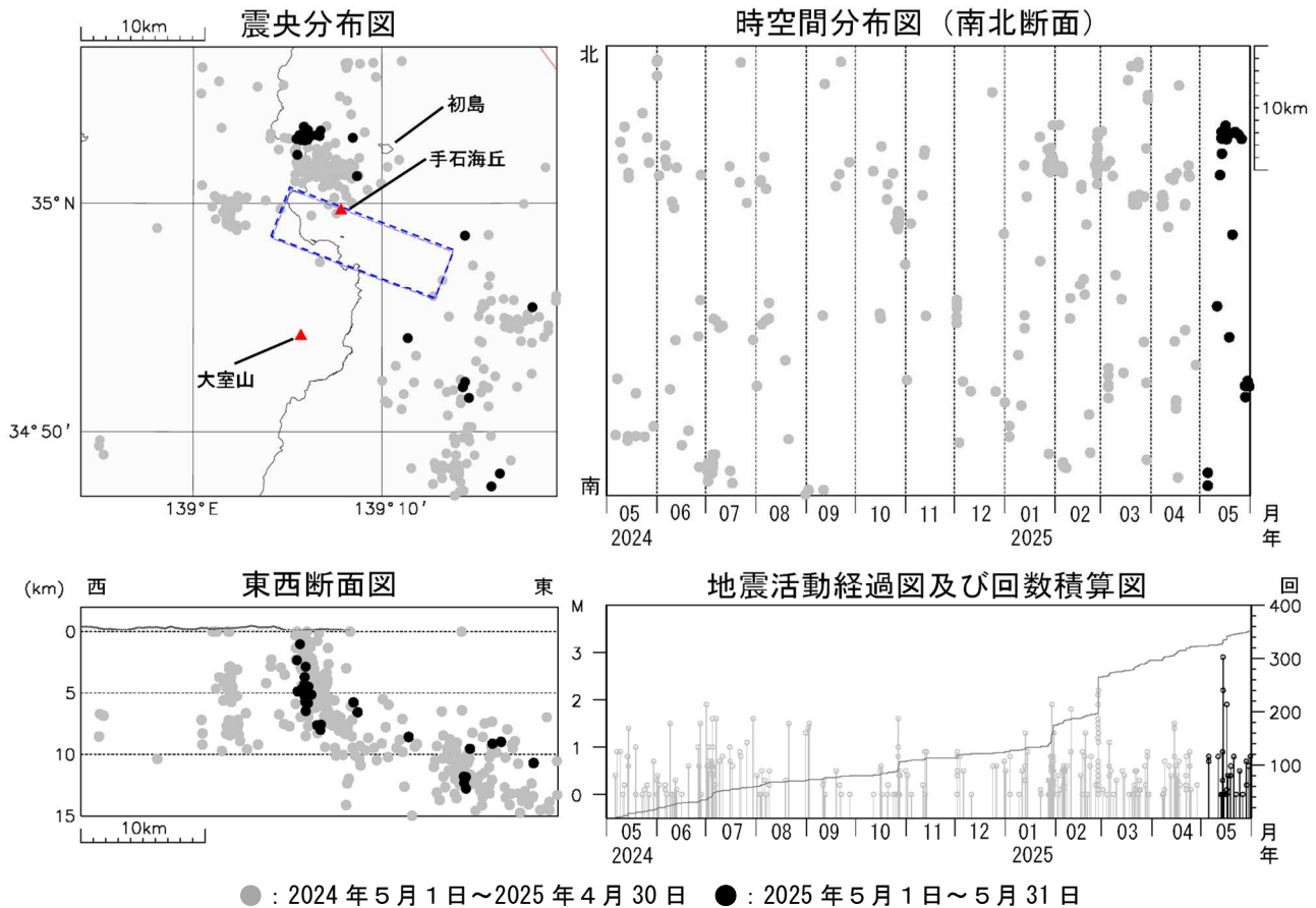
図2 伊豆東部火山群 広域地震観測網による震源分布図（2024 年 5 月 1 日～2025 年 5 月 31 日） □ の領域は群発地震活動の発生する可能性がある範囲（火口が出現する可能性のある範囲）を示しています。 https://www.data.jma.go.jp/vois/data/filing/level/PDF/level_316.pdf 広域地震観測網により震源決定したもので、深さは全て海面以下として決定しています。 M（マグニチュード）は地震の規模を表し、M0.0 以上を表示しています。 図中の震源要素は一部暫定値が含まれており、後日変更することがあります。 この図では、関係機関の地震波形を一元的に処理し、地震観測点の標高を考慮する等した手法で得られた震源を用いています。
