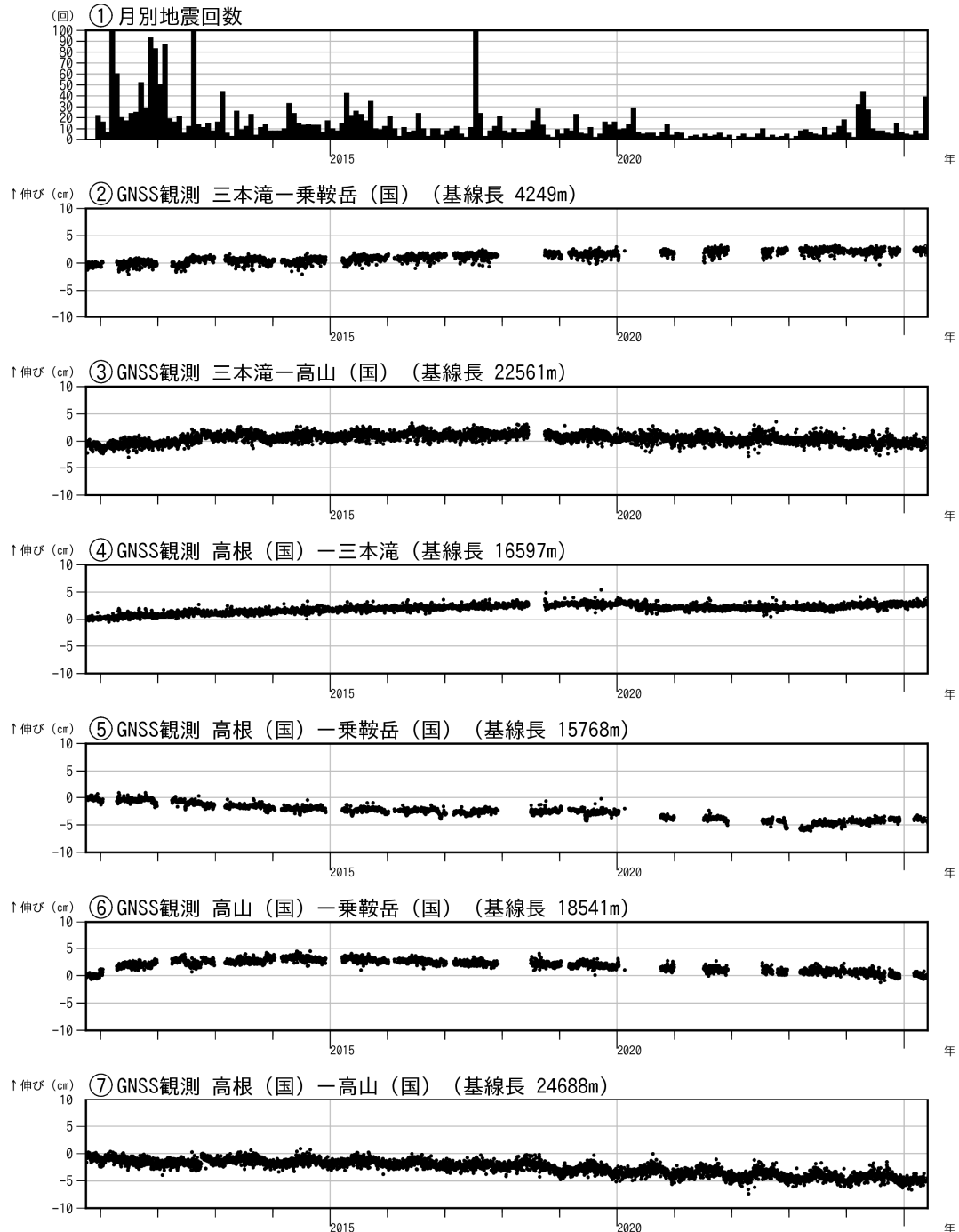
図2 乗鞍岳 火山活動経過図（2010年10月1日～2025年5月31日）
