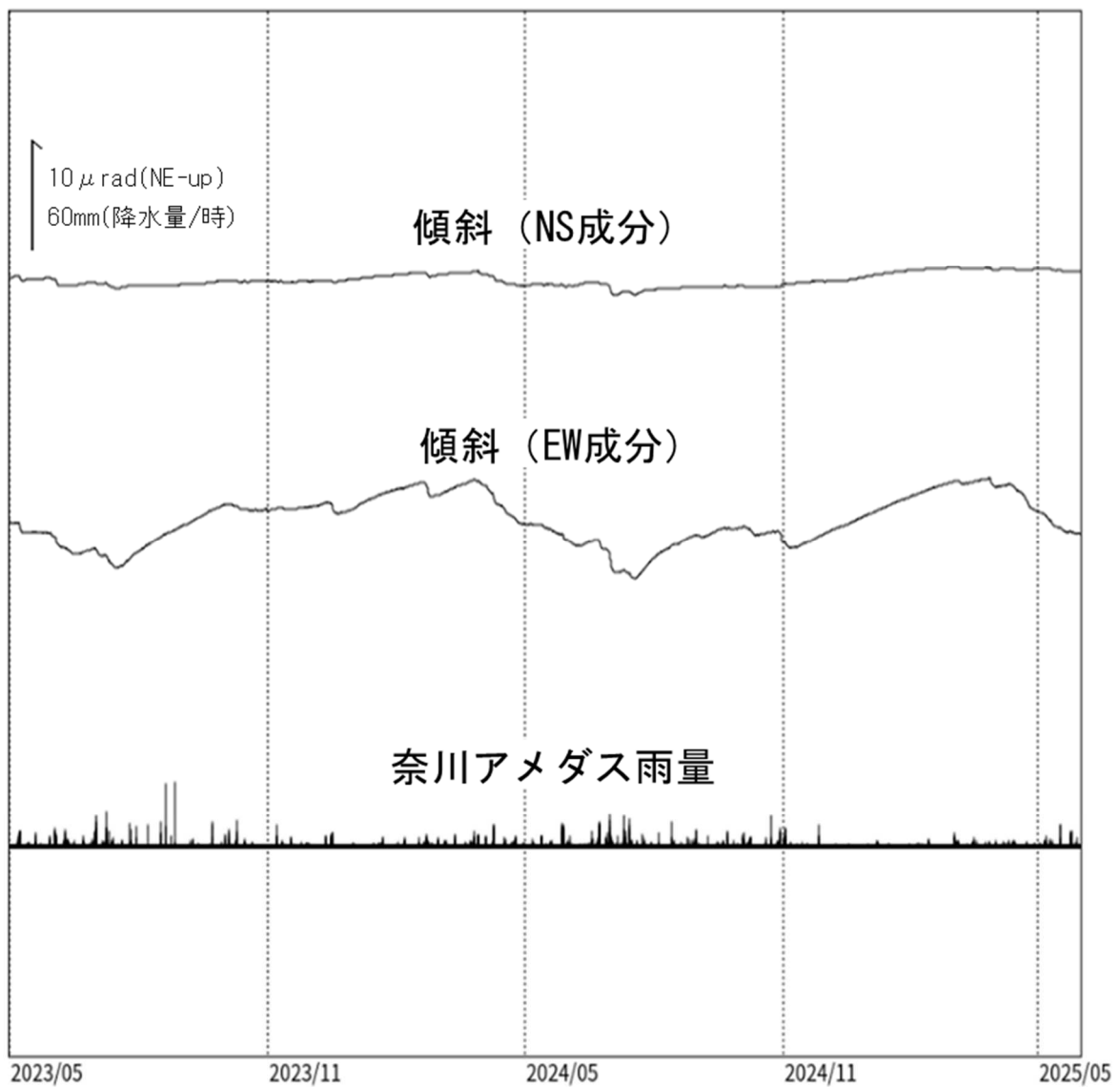
図4 乗鞍岳 三本滝観測点における傾斜データ（2023年5月1日～2025年5月31日）
