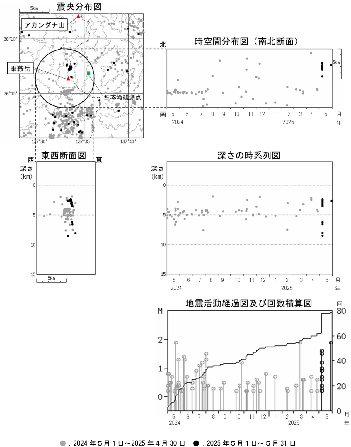
図3 乗鞍岳 広域地震観測網による山体・周辺の地震活動(2024年5月1日～2025年5月31日)
