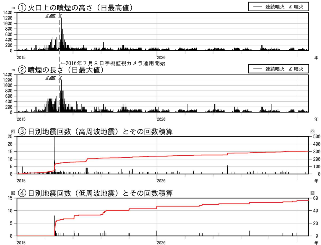
図3 新潟焼山 火山活動経過図（短期）（2015年1月1日～2025年5月31日）
