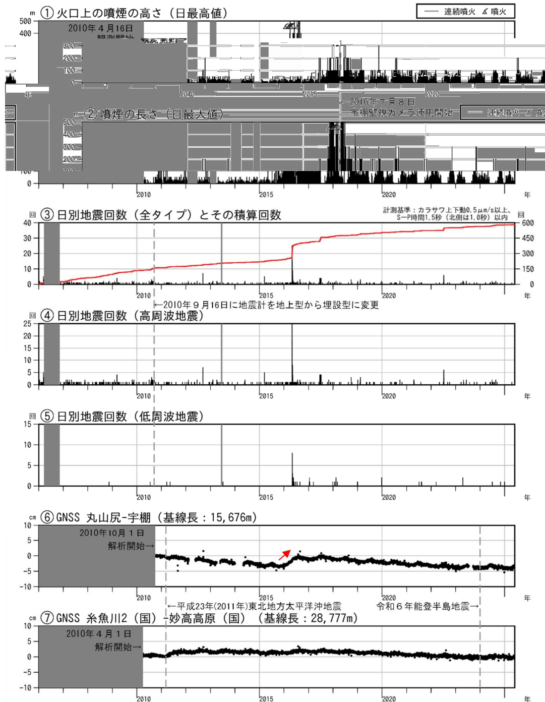
図2 新潟焼山 火山活動経過図（2006年1月1日～2025年5月31日）
