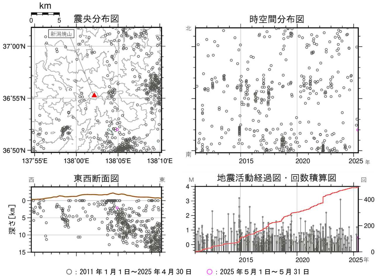
図 4 新潟焼山 広域地震観測網による山体・周辺の地震活動（2011 年 1 月 1 日～2025 年 5 月 31 日）
