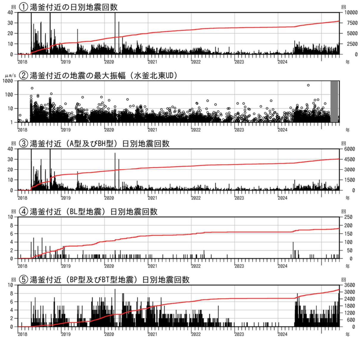
図 1 - 1 草津白根山（白根山（湯釜付近）） 湯釜付近の地震活動の状況 (2018 年 1 月 1 日～2025 年 5 月 31 日)
