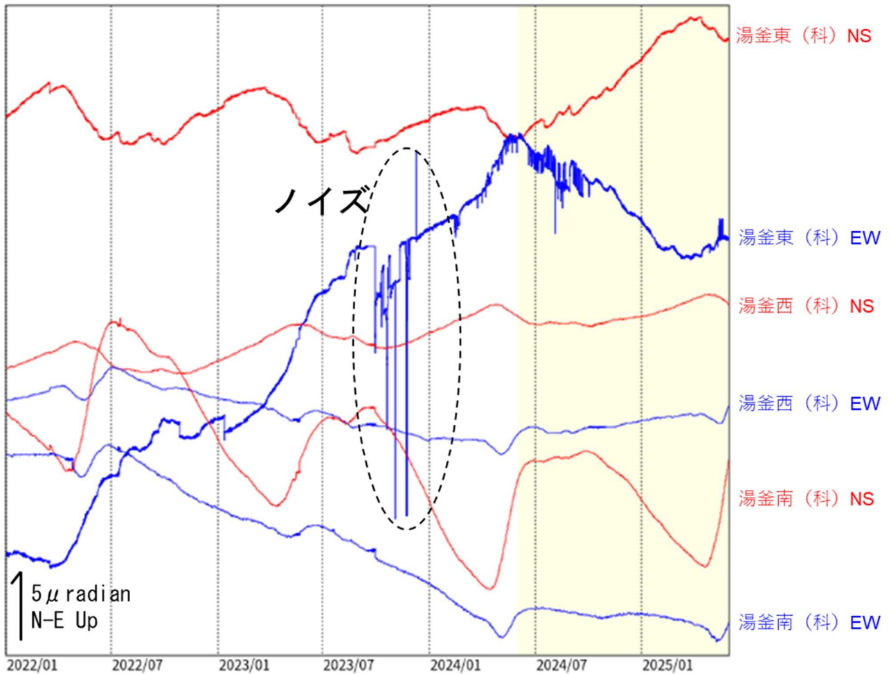
図5 草津白根山（白根山（湯釜付近）） 傾斜変動（2022年1月1日～2025年5月31日） データは時間平均値を使用しています。（科）：東京科学大学
