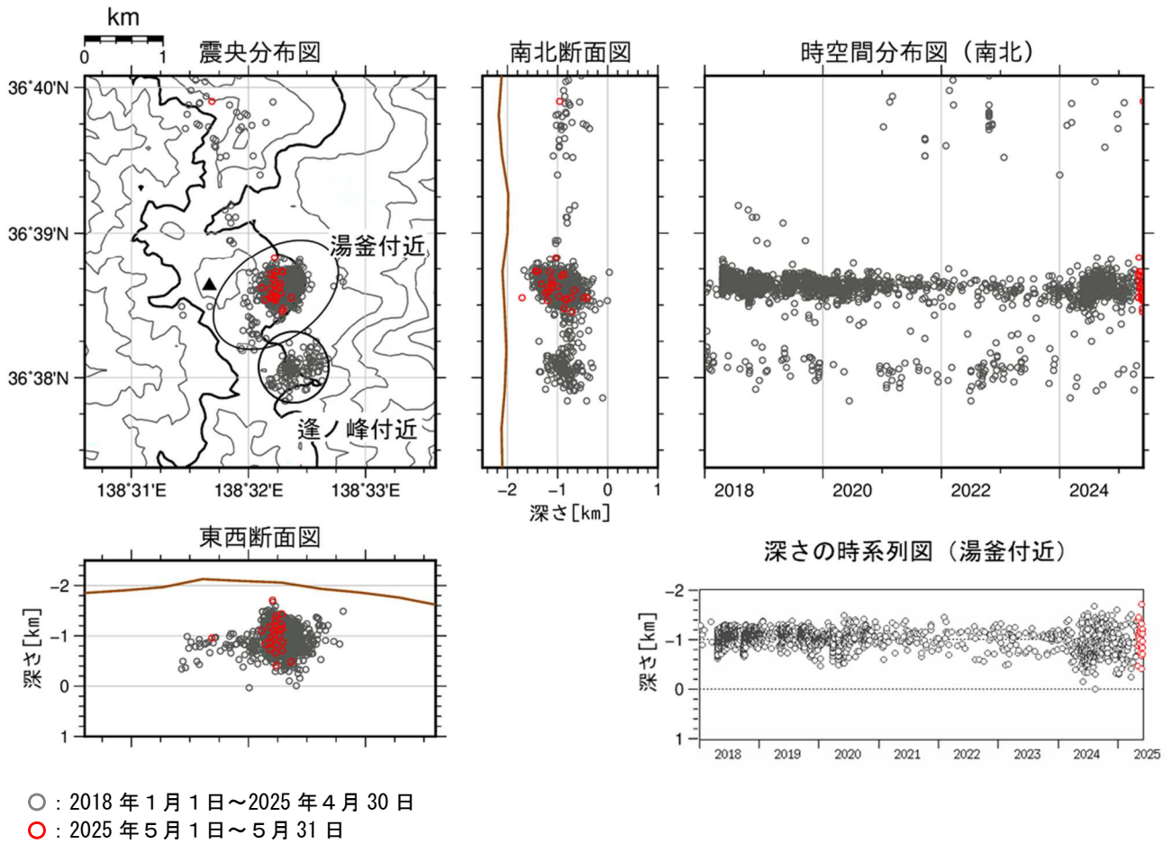
図4 草津白根山 震源分布図（2018 年 1 月 1 日～2025 年 5 月 31 日）
