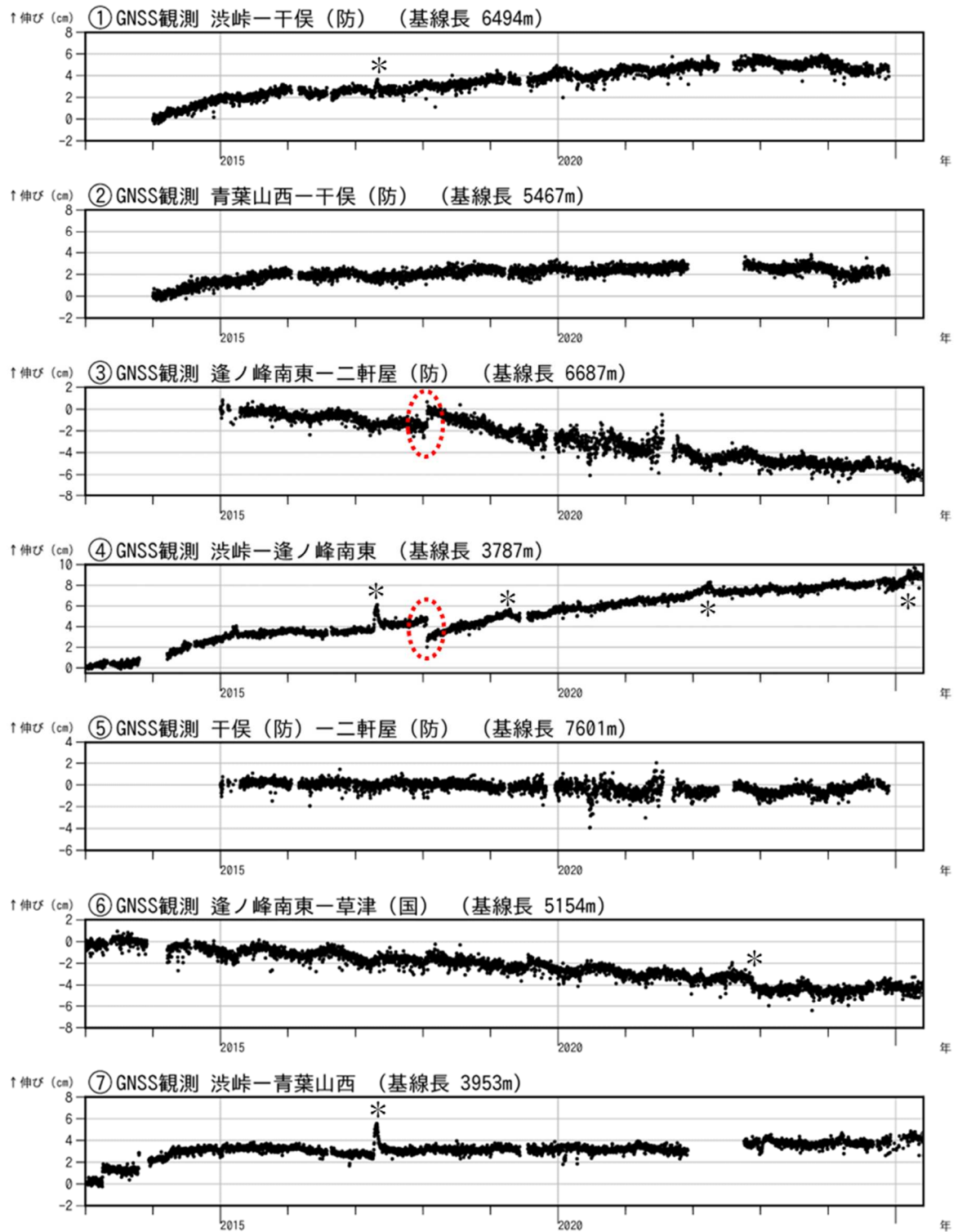
図6 草津白根山 GNSS 連続観測の結果（2013 年 1 月 1 日～2025 年 5 月 31 日）
