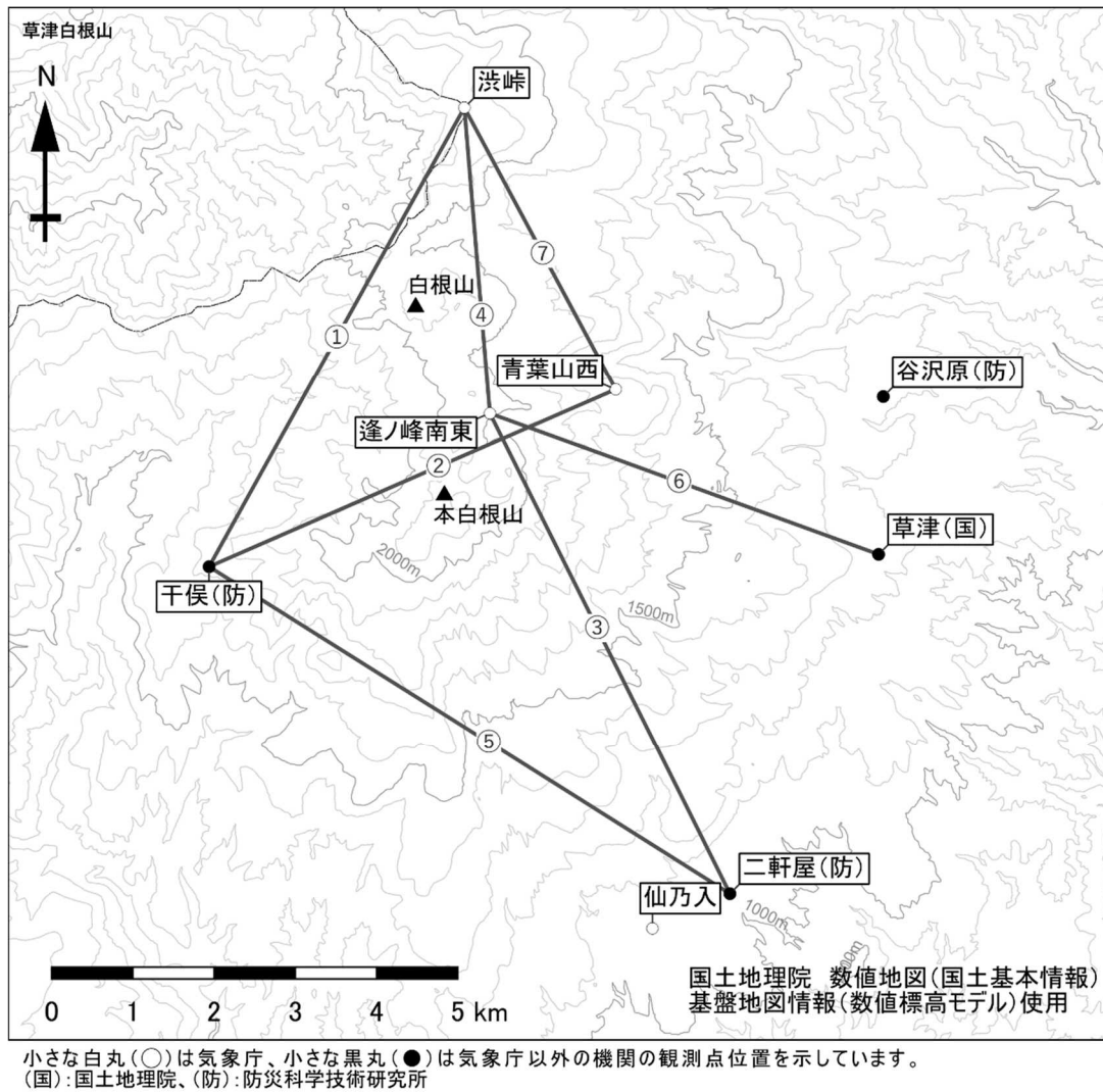
図7 草津白根山 GNSS 観測点配置図
