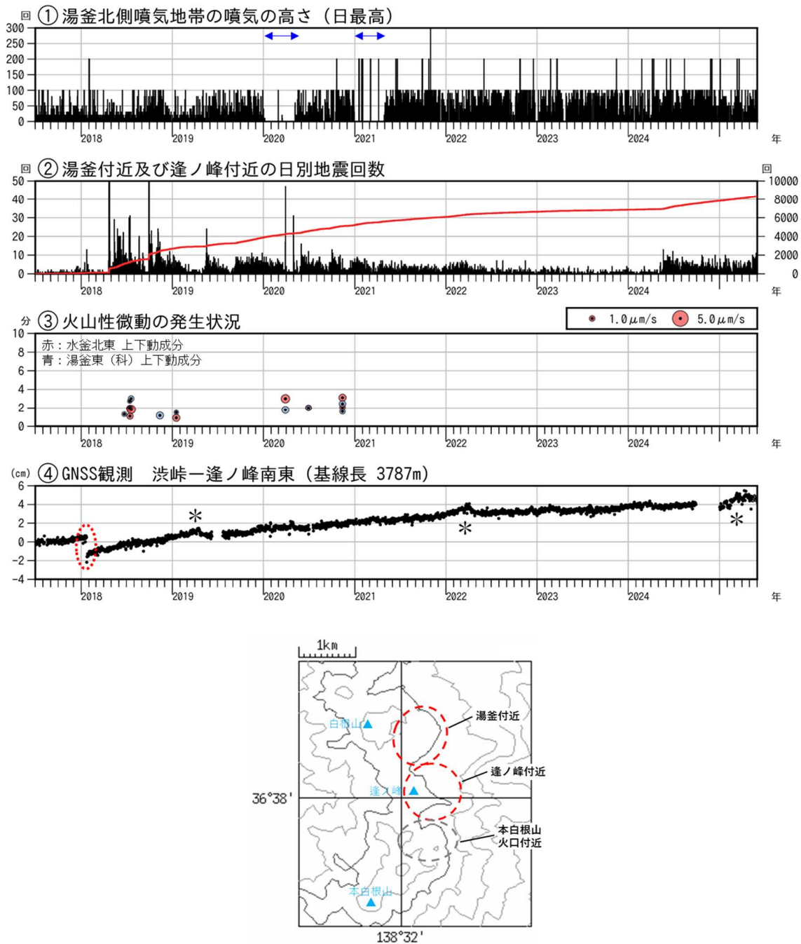
図3 草津白根山（白根山（湯釜付近）） 火山活動経過図（2017年7月1日～2025年5月31日）
