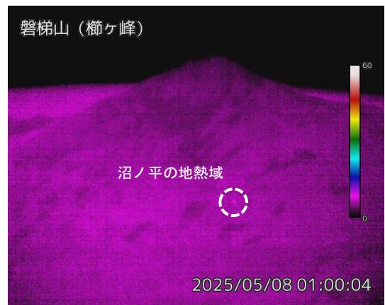
図2 磐梯山 沼ノ平周辺の状況（5月10日）と地表面温度分布（5月8日）
