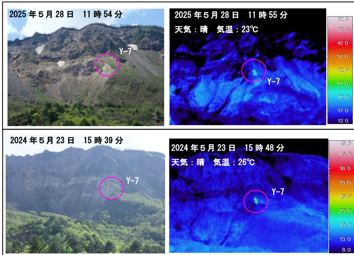
図 5 磐梯山 山体北側火口壁噴気地帯（Y-7）の状況（左）と地表面温度分布（右）
