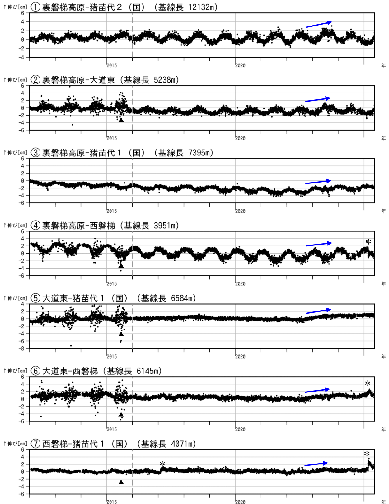
図 10 磐梯山 GNSS 基線長変化図 (2012 年 1 月～2025 年 5 月)
