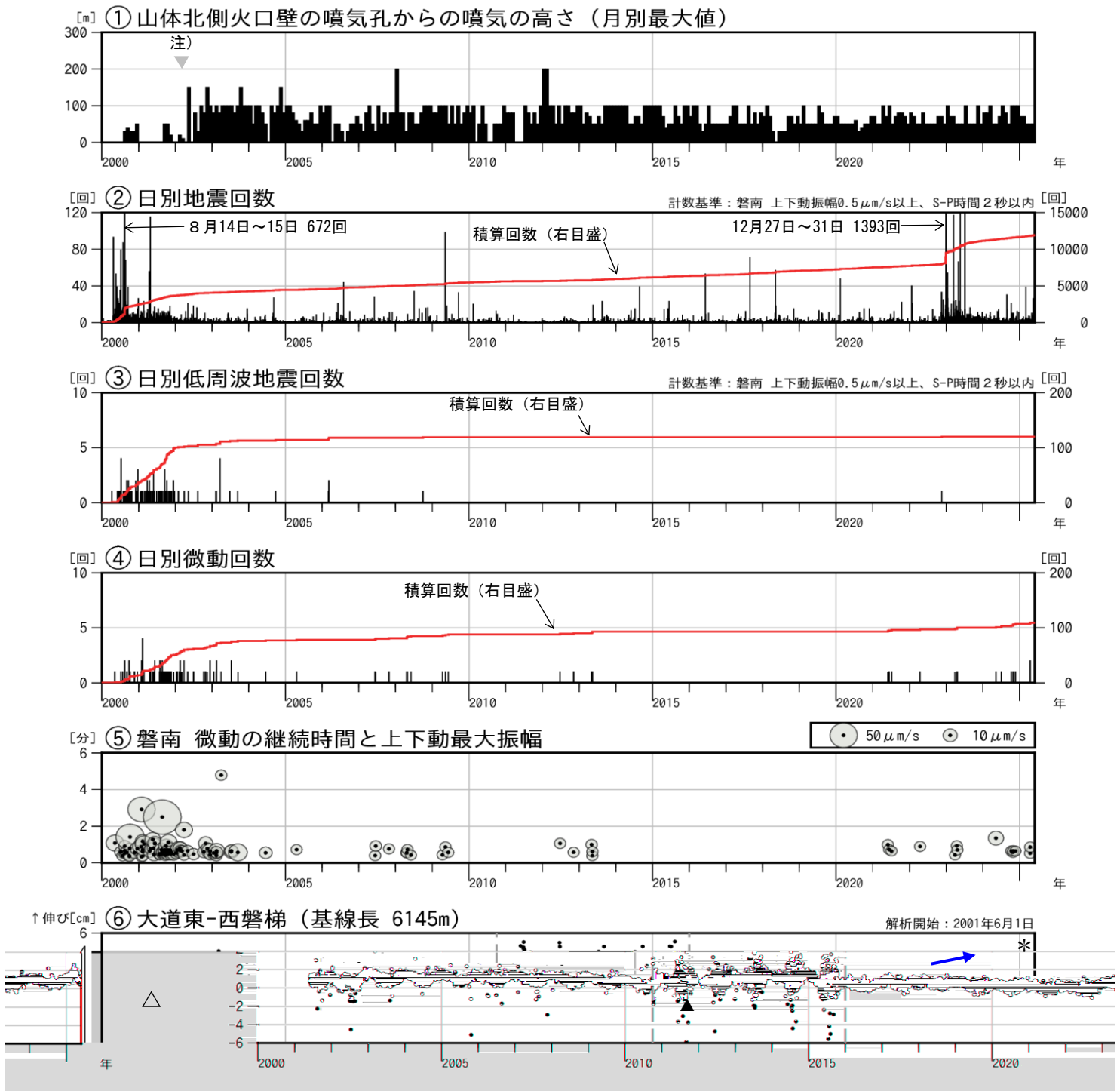
図7 磐梯山 火山活動経過図（2000年1月～2025年5月）
