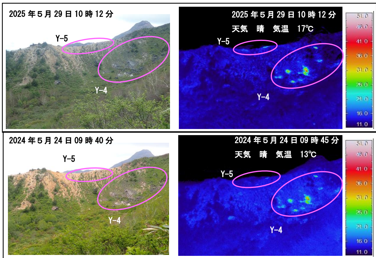
図 6 磐梯山 山体北側火口壁噴気地帯（Y-4、Y-5）の状況（左）と地表面温度分布（右）
