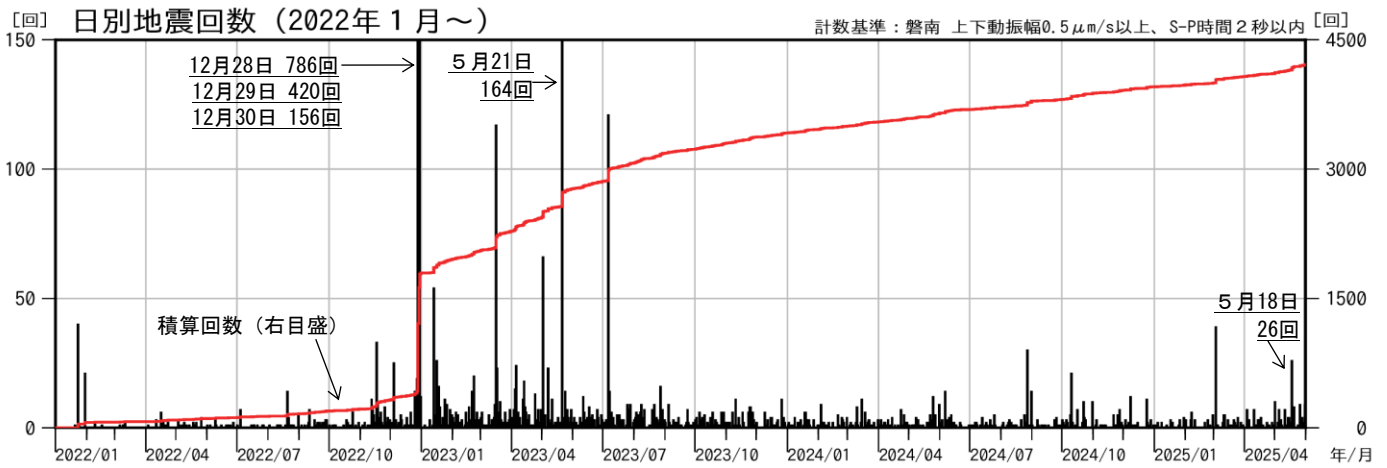
図8 磐梯山 地震回数（2022年1月～2025年5月）
