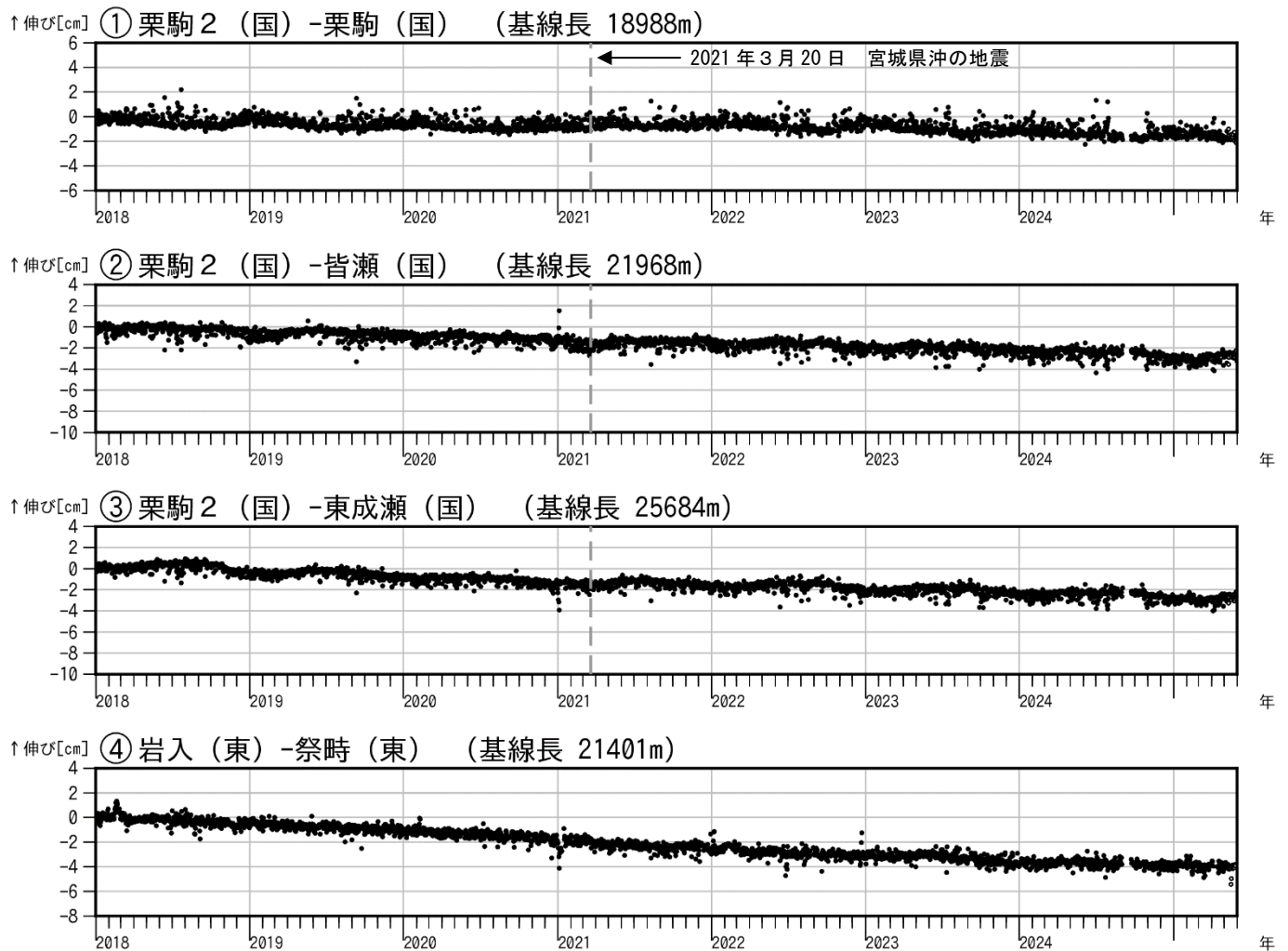
図3 栗駒山 GNSS 基線長変化図（2018年1月～2025年5月）
