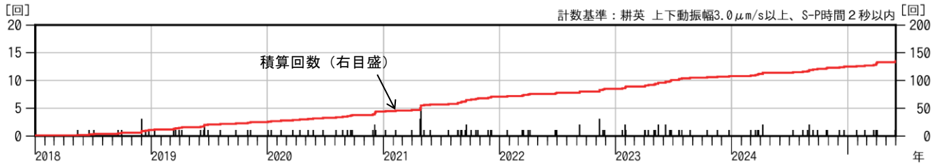
図2 栗駒山 日別地震回数（2018年1月～2025年5月）
