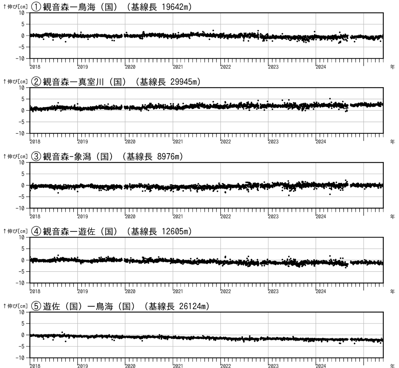
図4 鳥海山 GNSS 基線長変化図（2018年1月～2025年5月）
