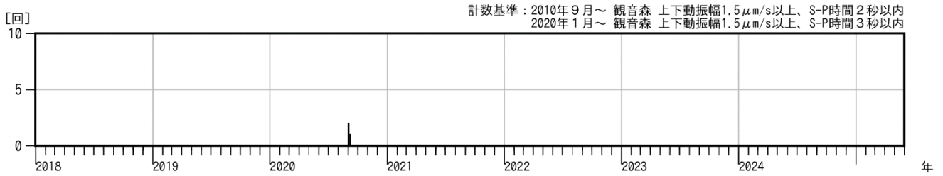
図3 鳥海山 火山性地震の日別回数（2018年1月～2025年5月）
