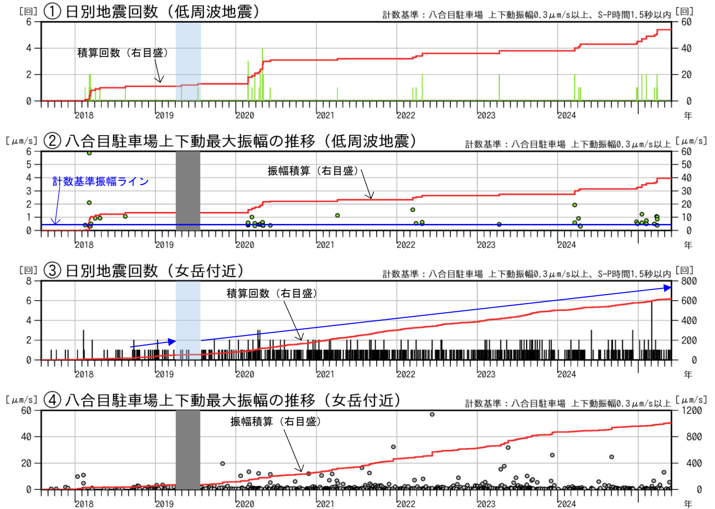
図2 秋田駒ヶ岳 低周波地震及び女岳付近の日別回数と最大振幅（2017年8月～2025年5月）
