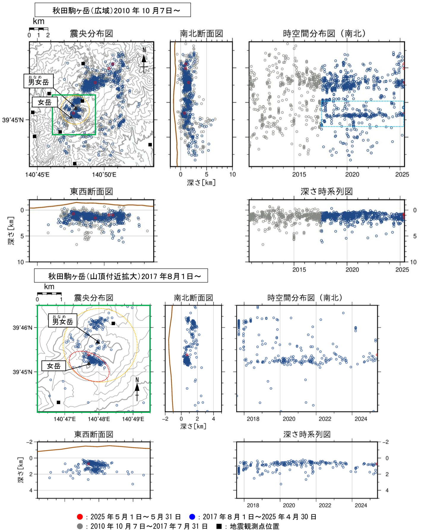
図3 秋田駒ヶ岳 地震活動（2010年10月7日～2025年5月）
