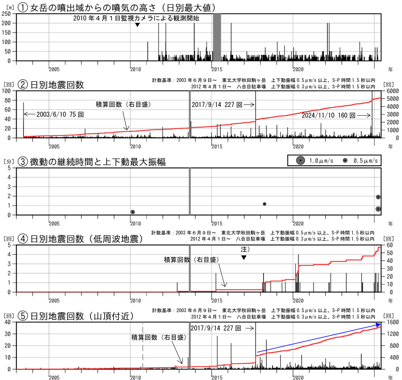
図 1 秋田駒ヶ岳 火山活動経過図（2003 年 6 月～2025 年 5 月）
