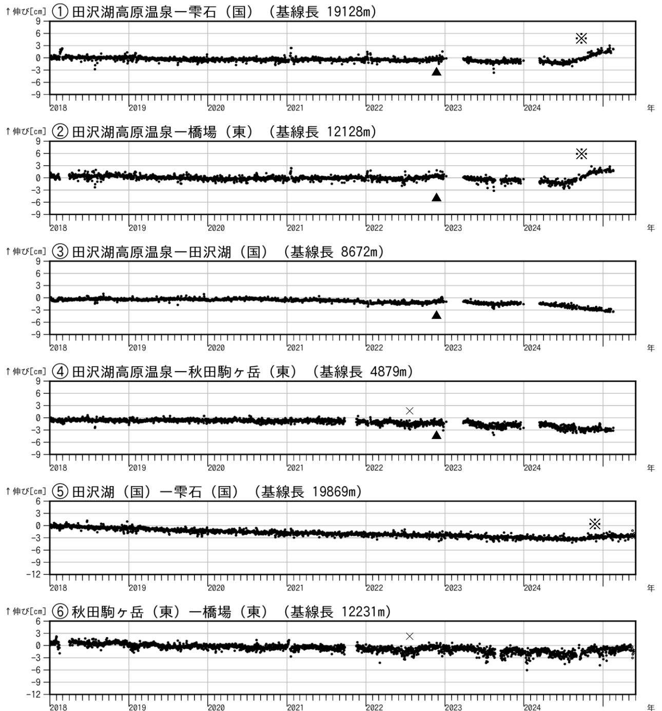
図4 秋田駒ヶ岳 GNSS 基線長変化図（2018年1月～2025年5月）
