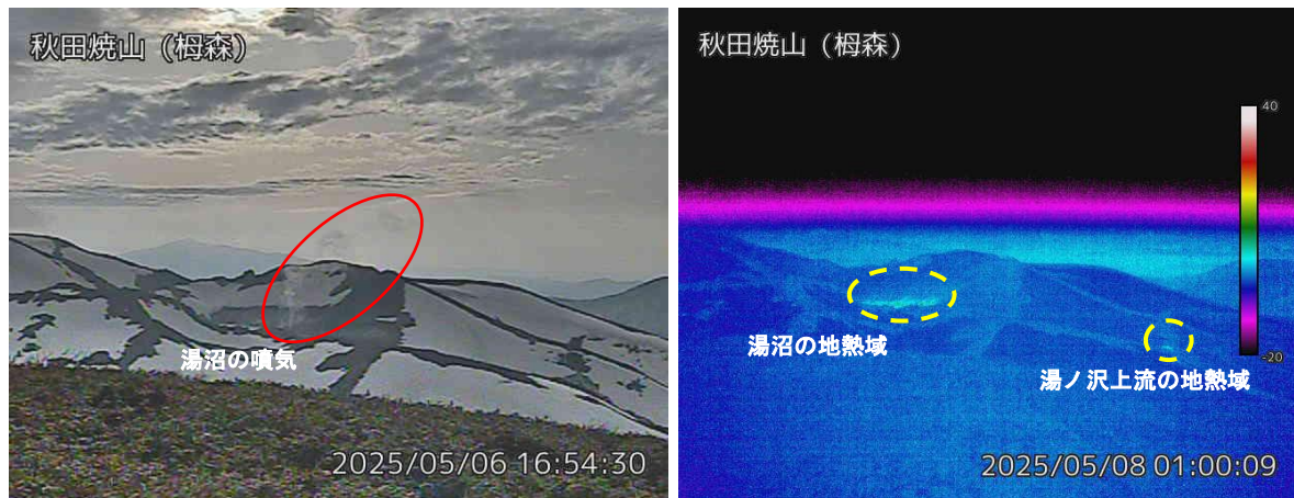
図2 秋田焼山 湯沼と湯ノ沢上流の状況（5月6日）と地表面温度分布（5月8日）
