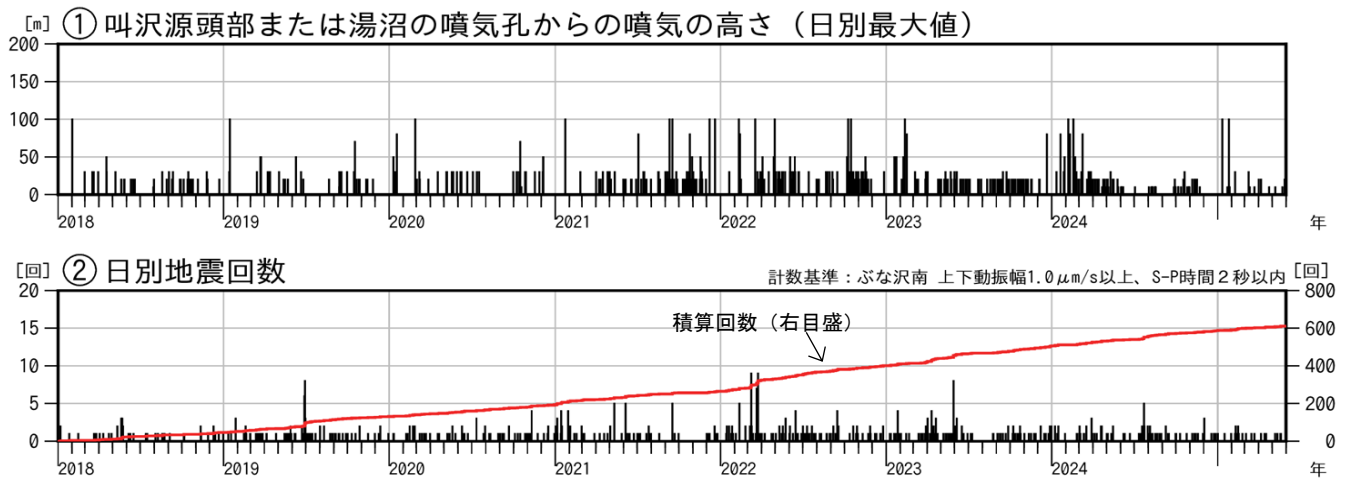
図3 秋田焼山 火山活動経過図（2018年1月～2025年5月）
