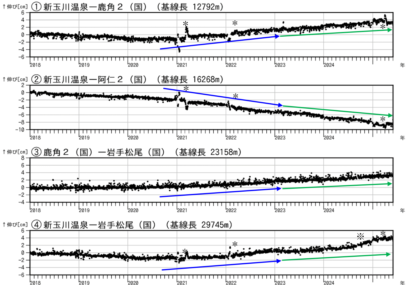
図4 秋田焼山 GNSS 基線長変化図（2018年1月～2025年5月）
