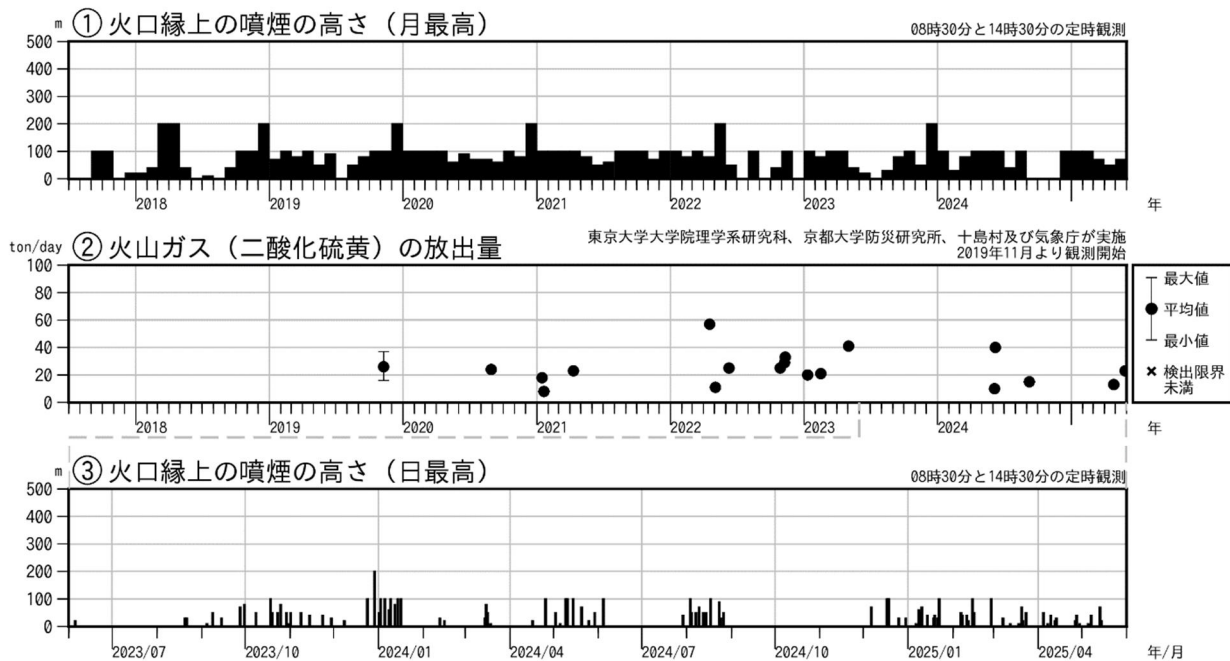
図2 中之島 火山活動経過図（2017年7月～2025年5月）
