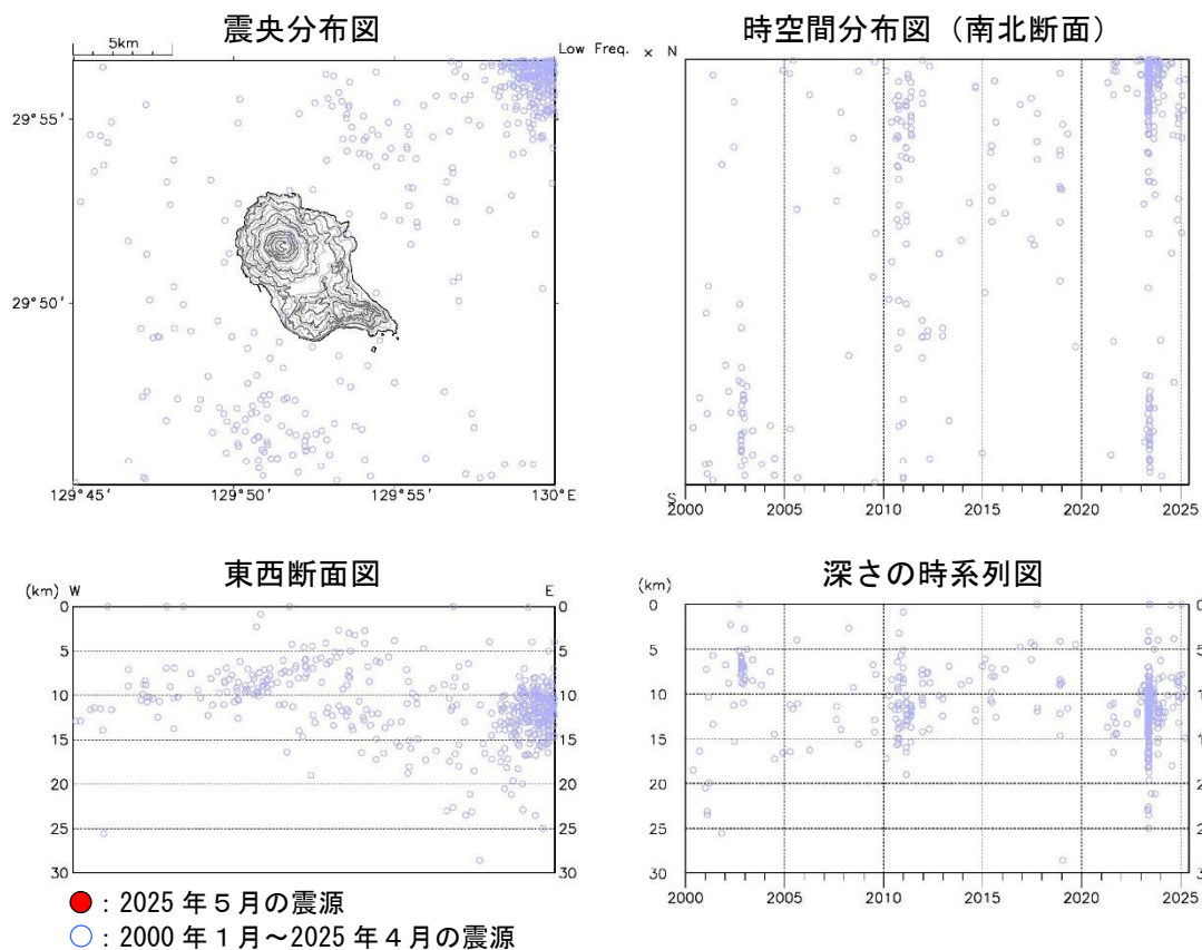
図3 中之島 中之島周辺の震源分布図（2000年1月～2025年5月）
