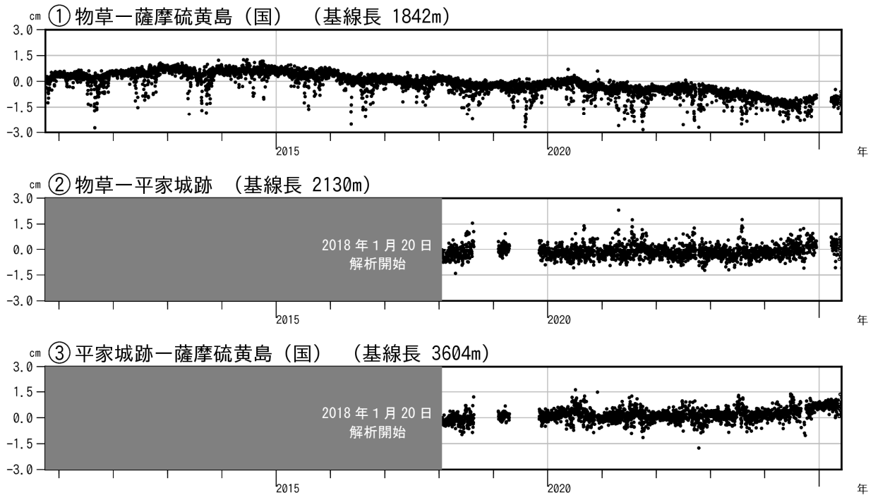
図5 薩摩硫黄島 GNSS連続観測による基線長変化（2010年10月～2025年5月）
