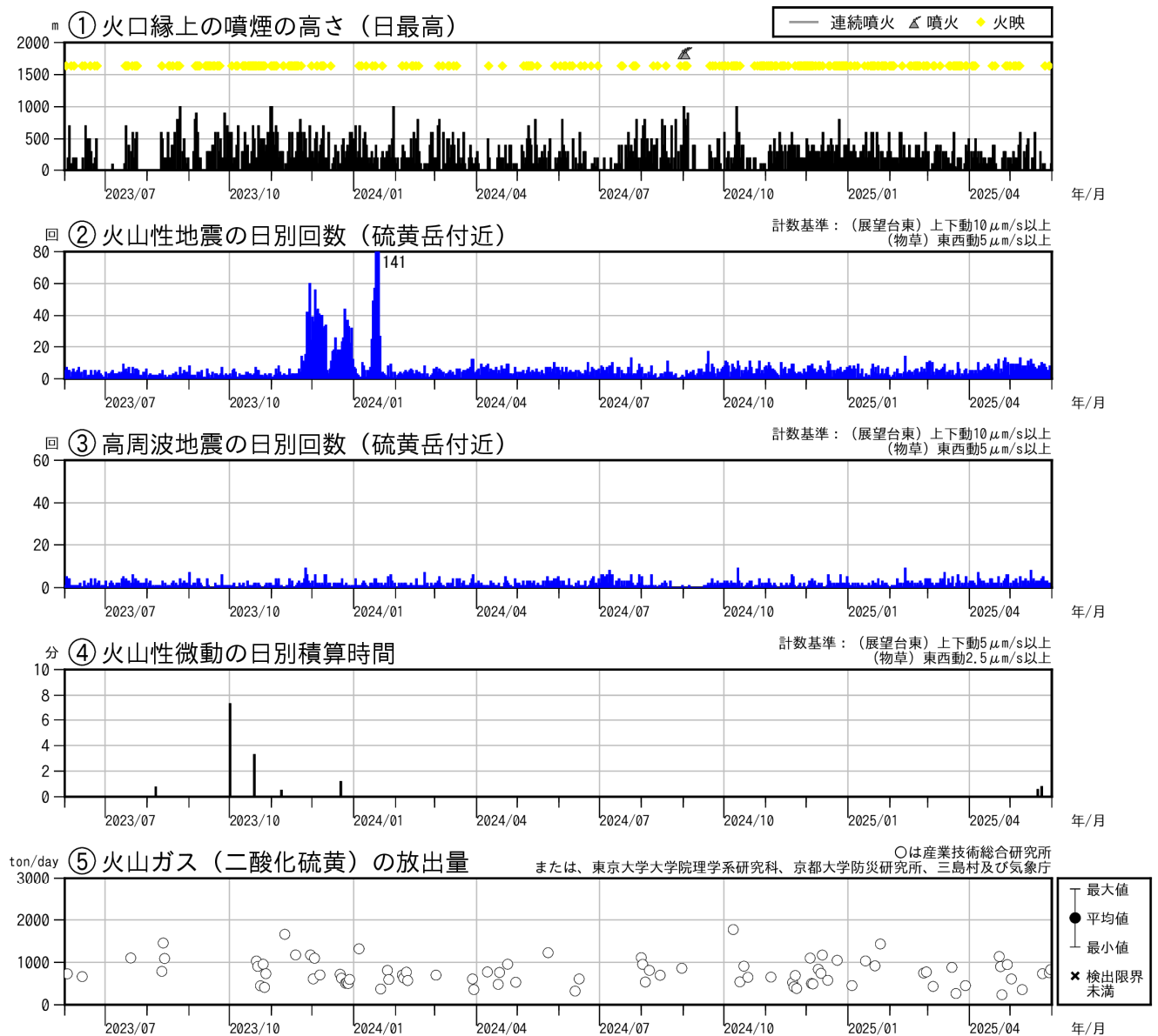
図3 薩摩硫黄島 火山活動経過図（2023年6月～2025年5月）
