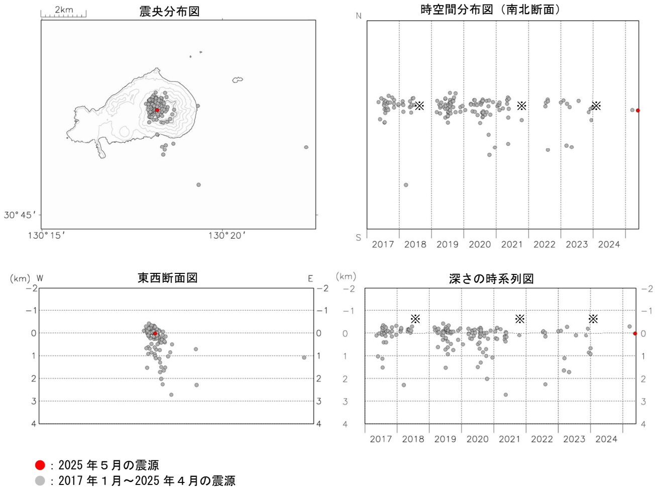
図4 薩摩硫黄島 火山性地震の震源分布図（2017 年 1 月～2025 年 5 月）
