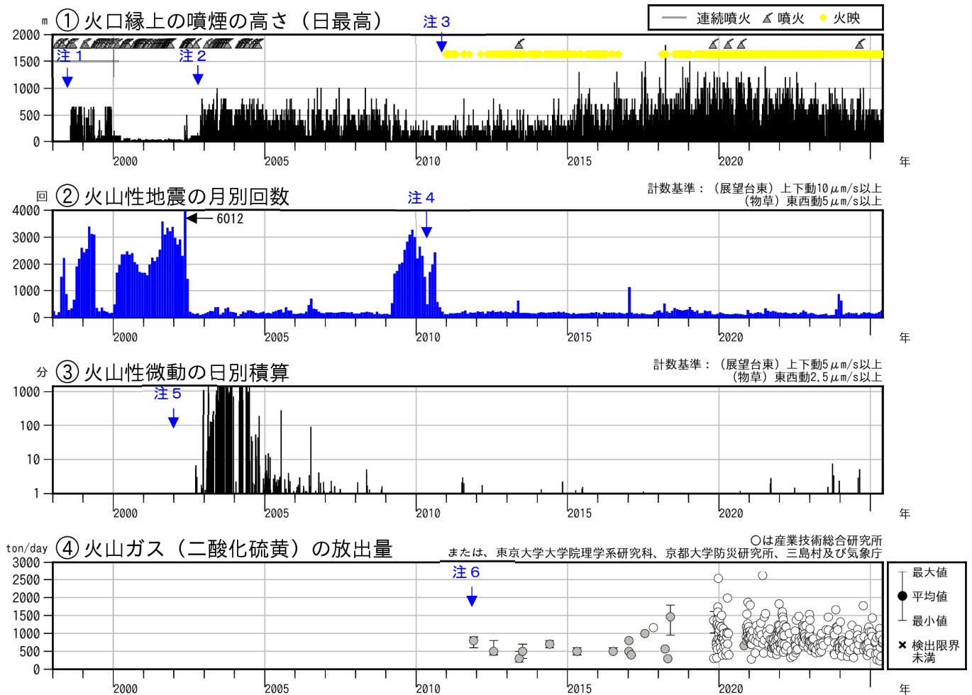
図2 薩摩硫黄島 火山活動経過図（1998年1月～2025年5月）
