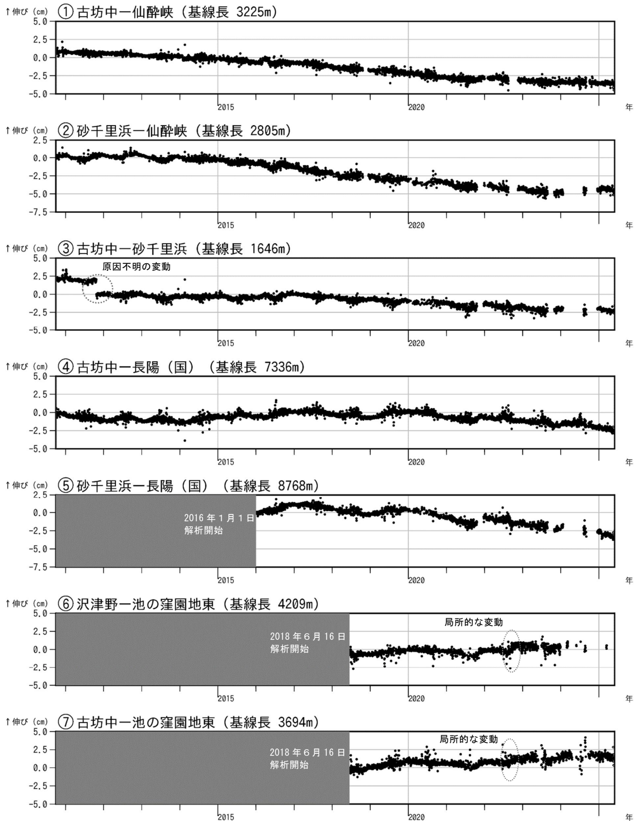
図 6 阿蘇山 GNSS 連続観測による基線長変化（2010 年 10 月～2025 年 5 月）
