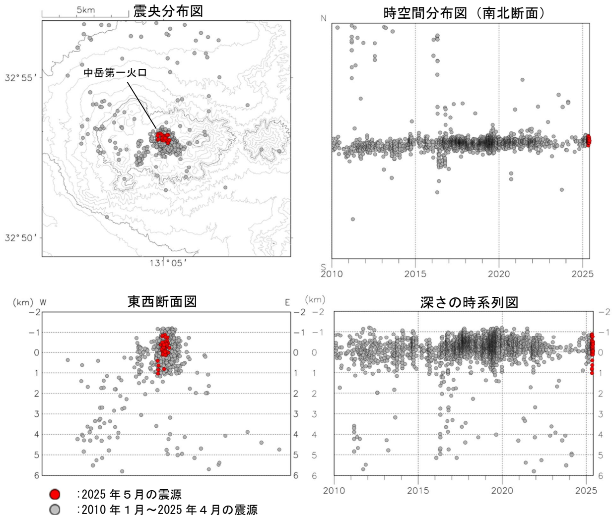
図5 阿蘇山 火山性地震の震源分布
